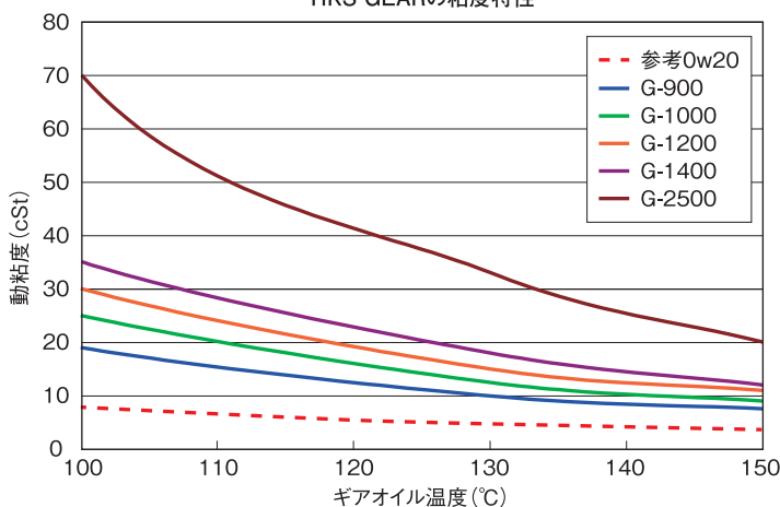
HKS GEARの粘度特性
